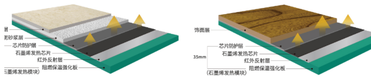
石墨烯发热模块结构图
